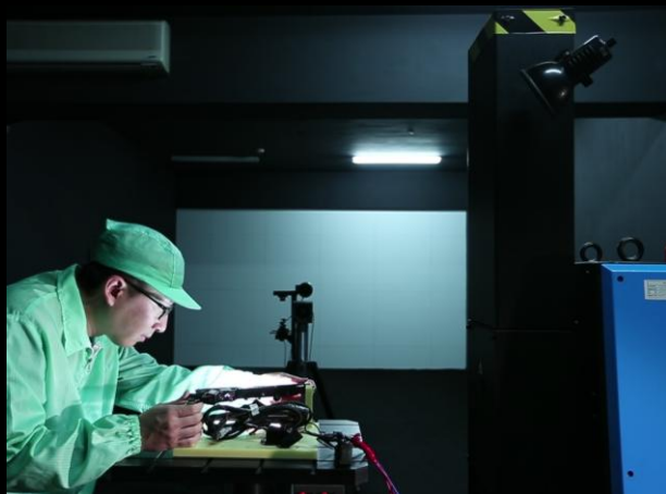
Goniophotometer Lab 配光實驗室
